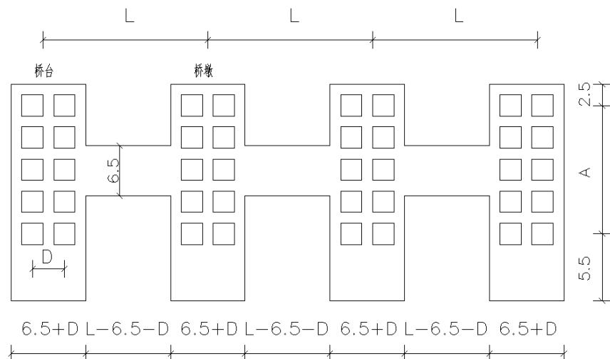
工作平台面积计算 单位：m 2
