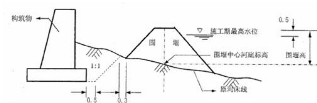
围堰剖面示意图 单位：m
