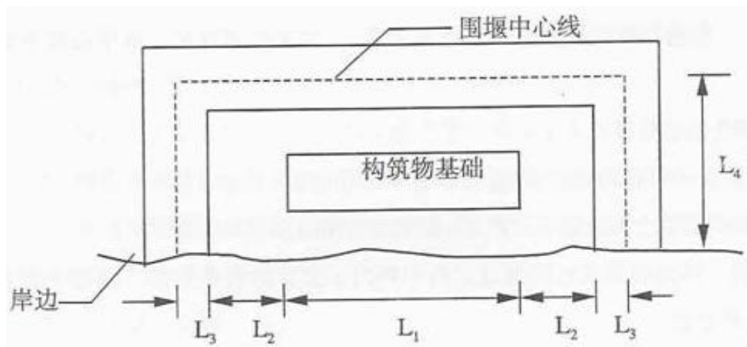
围堰平面示意图
