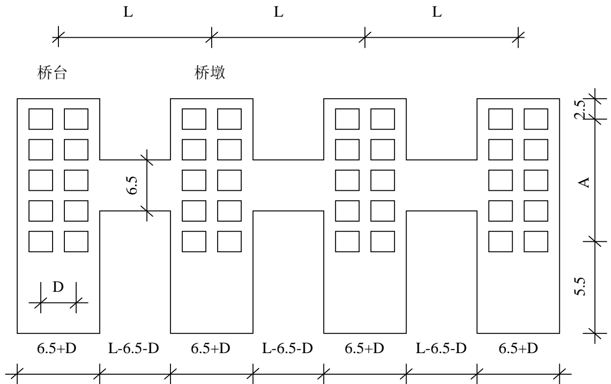
图 3.1.2 工作平台面积计算示意图
